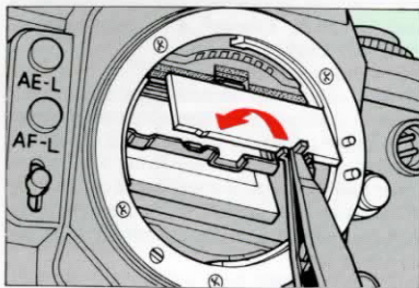
4. Placez soigneusement la nouvelle plage dans son châssis, à l'aide des pincettes en vérifiant que sa face plane est dirigée le bas.
