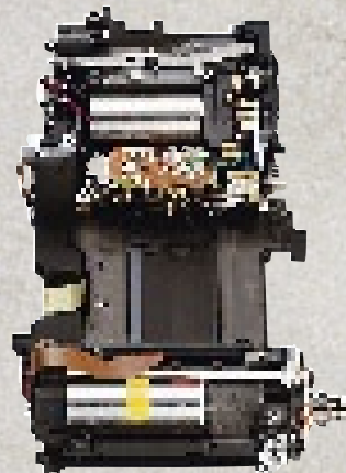
Châssis arrière : Rembobinage du film et contrôle de charge de l'obturateur
